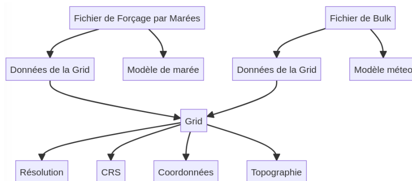
FIGURE 12 – Schéma de l'organisation des données pour le modèle CROCO.
